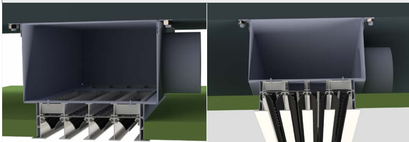
Монтаж диффузоров серии АДЛ
