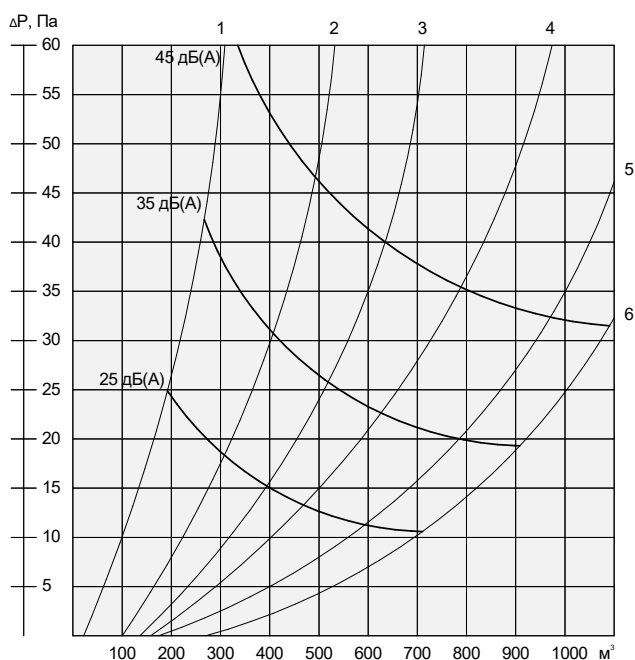
АДЛ-П, АДЛ-ПЗ угол наклона ламели \alpha = 0^\circ
