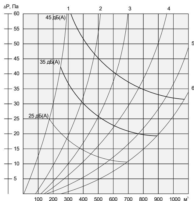
АДЛ-ПЗ угол наклона ламели \alpha = 30^\circ
