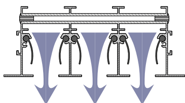
Прямоточная струя ( \alpha = 0^\circ )
