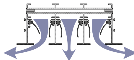
Разносторонняя струя ( \alpha = 0^\circ, \alpha = 50^\circ )
