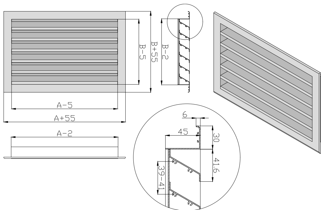
Габаритно-посадочные размеры фасадной решетки RH-40 AxB – размеры строительного проема
