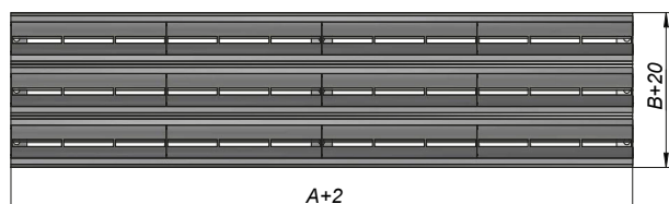
M Промежуточная секция
