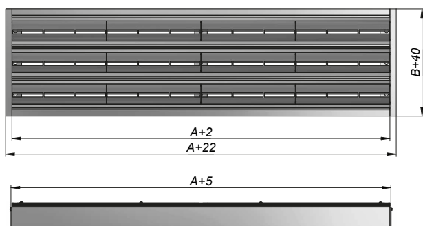
F1 Одиночная секция с фланцами
