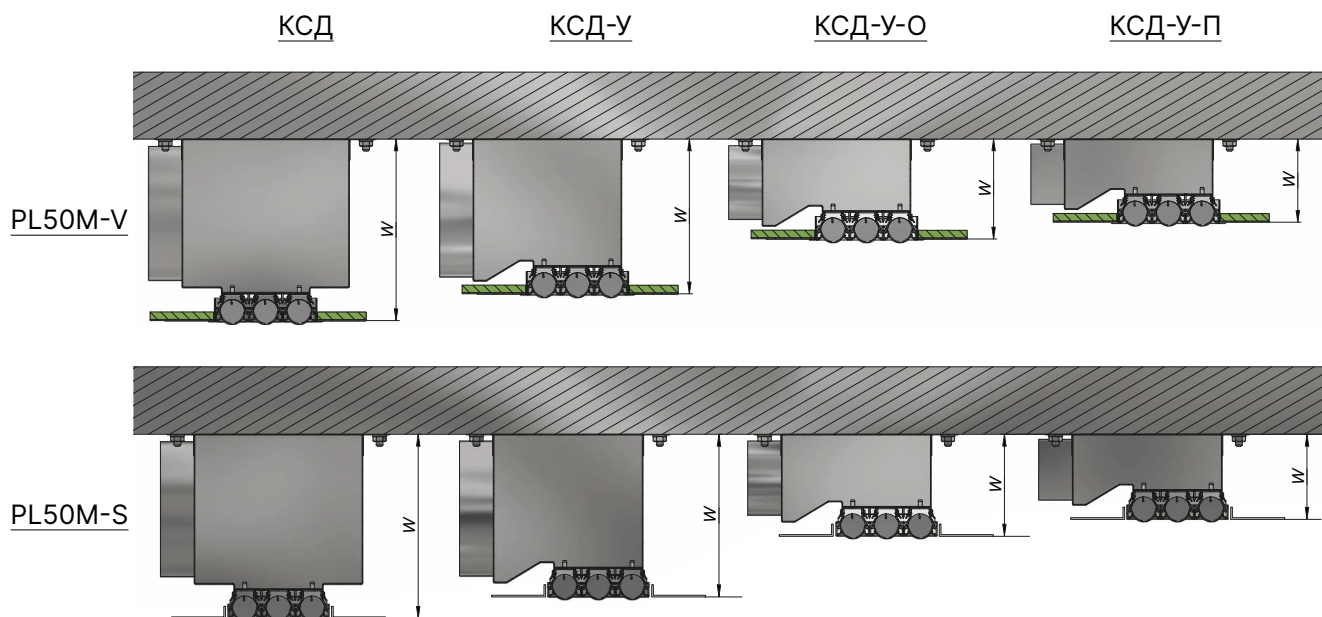
Размер монтажного пространства W min в зависимости от подводящего воздуховода
