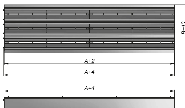
E2 Концевая секция с одной заглушкой
