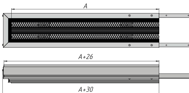
E2 Концевая секция с заглушкой
