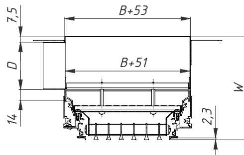
Сечение решетки
