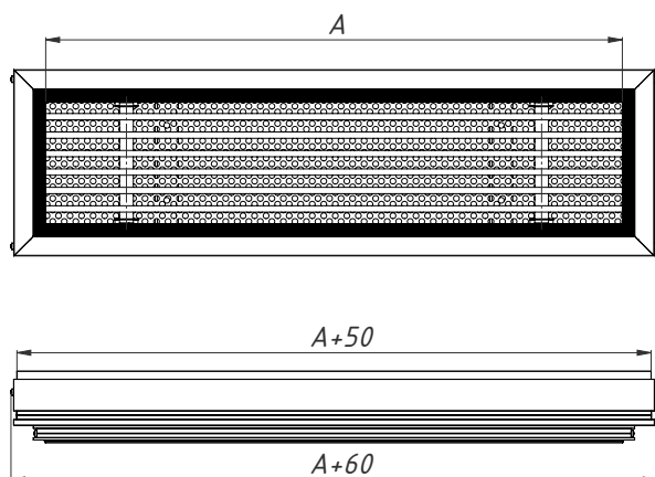
F1 Одиночная секция с фланцами
