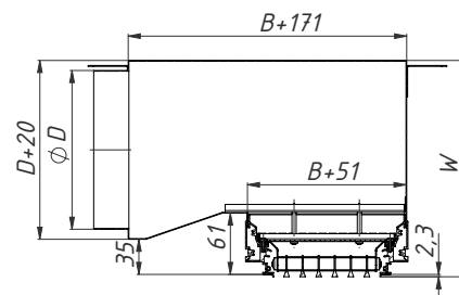
Сечение решетки
