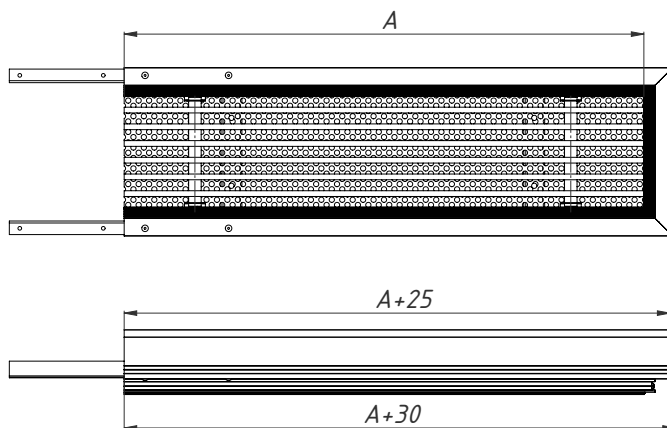
E1 Концевая секция с фланцем
