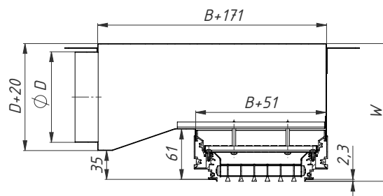
Сечение решетки
