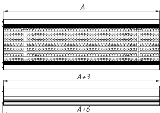
F2 Одиночная секция с заглушками
