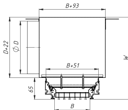
Сечение решетки
