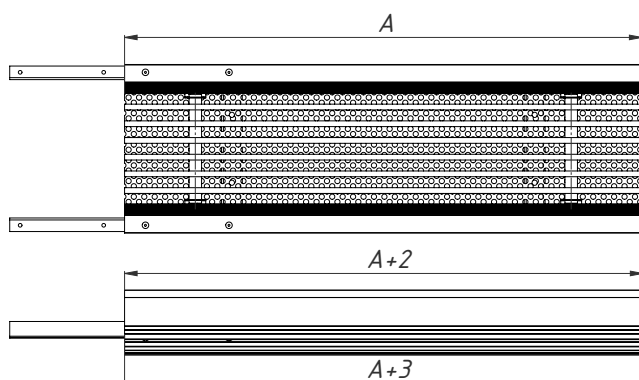
E2 Концевая секция с заглушкой
